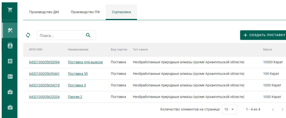
Рисунок 162 – Вкладка «Сортировка»
