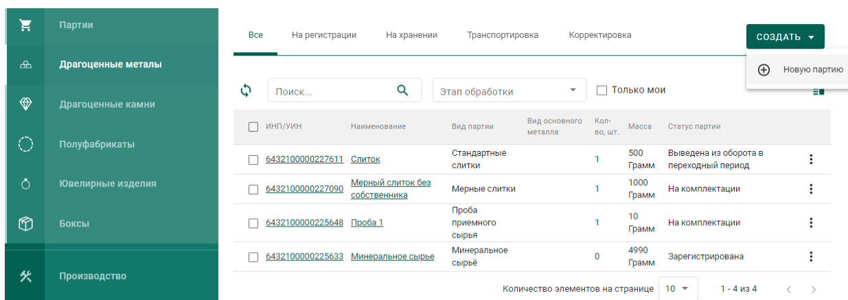
Рисунок 48 – Список партий
