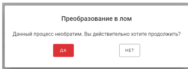
Рисунок 161 – Окно предупреждения
