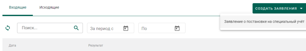
Рисунок 2 – Создание заявления
