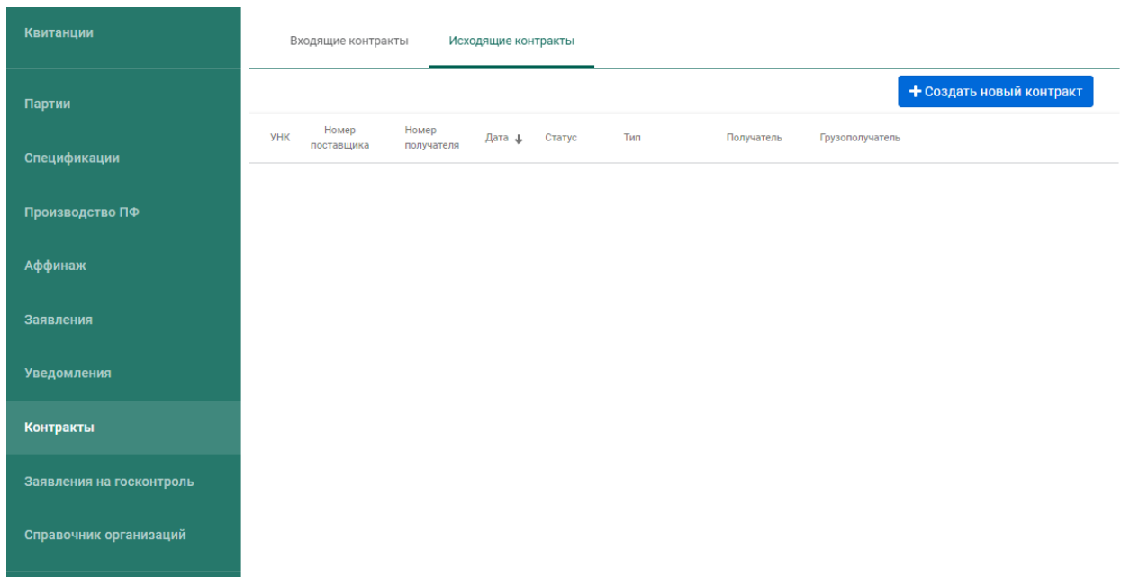
Рисунок 130 – Исходящие контракты
